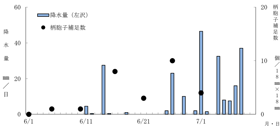
図1 降雨の状況と西洋なし輪紋病の柄胞子トラップによる飛散消長
